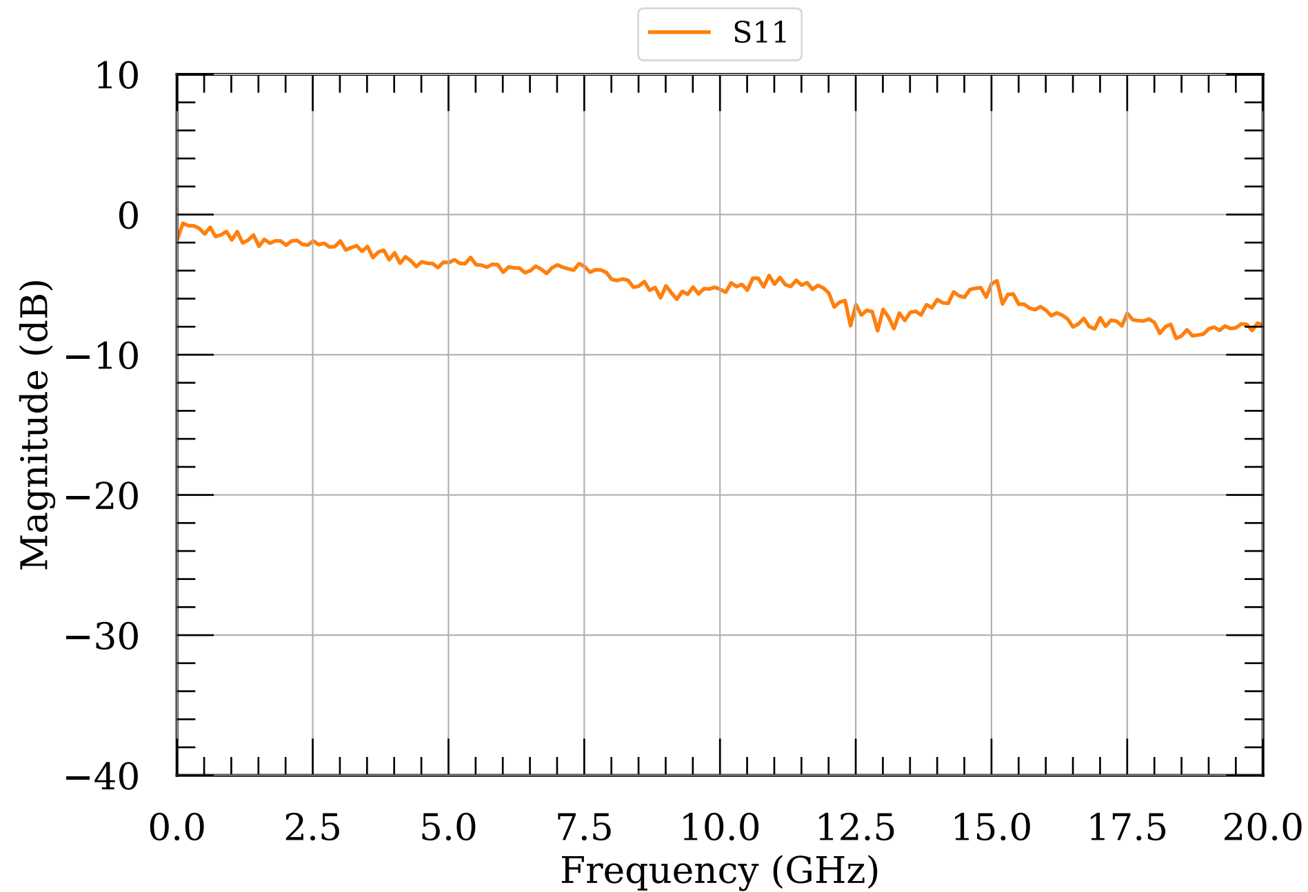
LNA S-params module040
